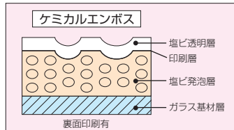
構造図
