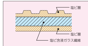
構造図
