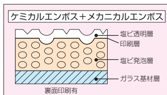
構造図
